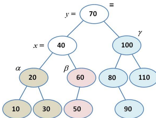
12.2. ábra. Az AVL-tulajdonság helyreállítása (++,+) forgatással
