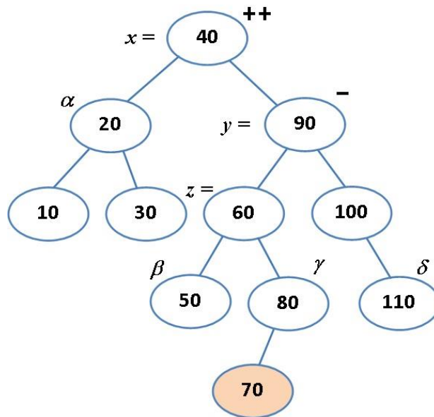
12.4. ábra. Az AVL-fa kiegyensúlyozottságának elomlása, (++)
