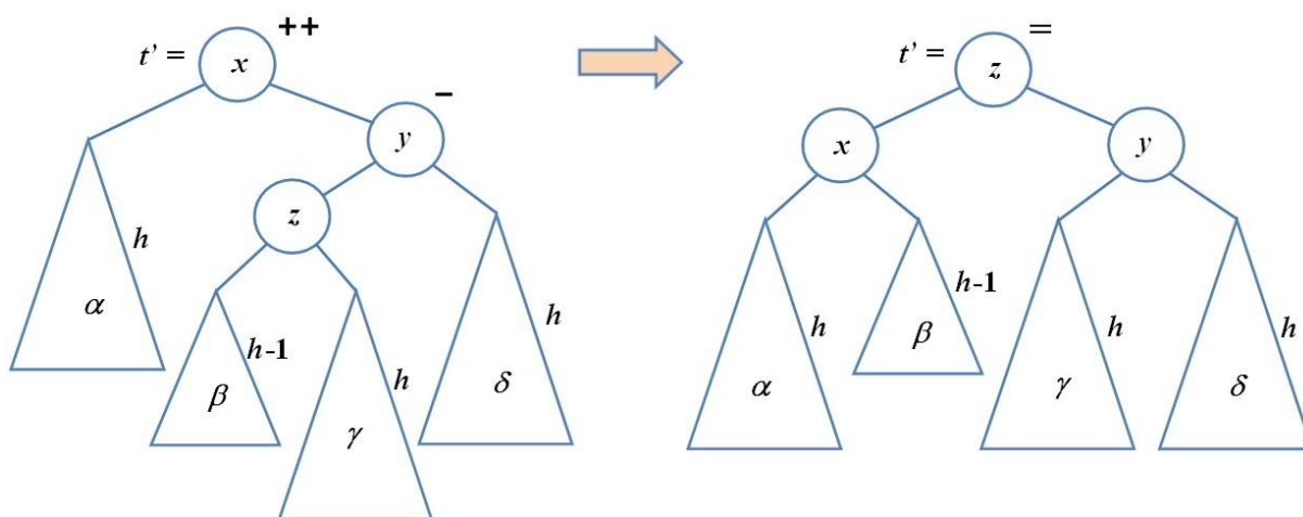
12.6. ábra. Az AVL-tulajdonság helyreállításának (+, -) sémája
