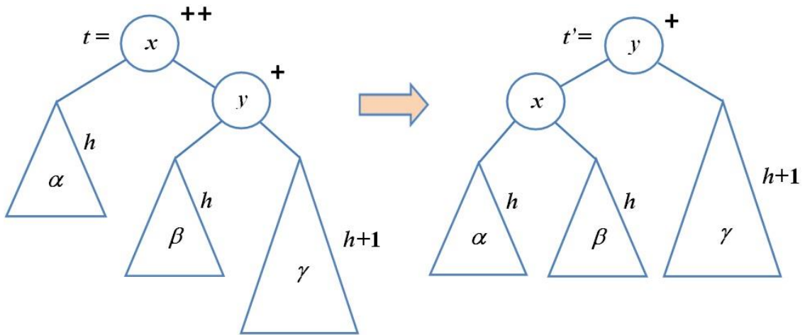
12.3. ábra. Az AVL-tulajdonság helyreállításának sémája, (++) eset
