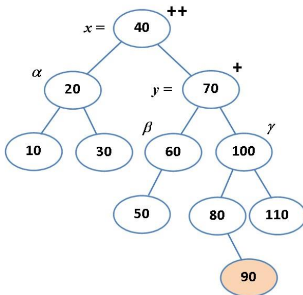
12.1. ábra. Az AVL-fa kiegyensúlyozottságának elromlása, (++,+) eset
