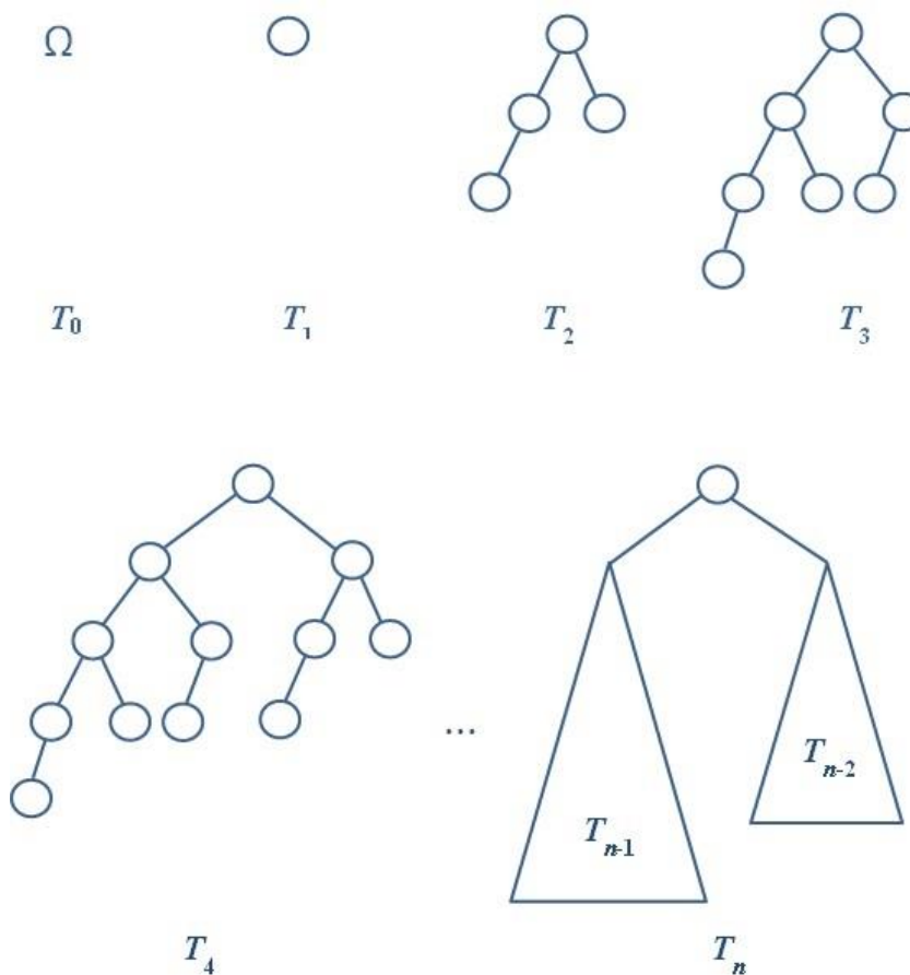
12.7. ábra. Fibonacci-fák
