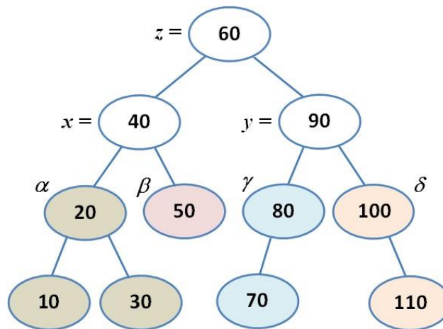
12.5. ábra. Az AVL-tulajdonság helyreállítása (++) forgatással
