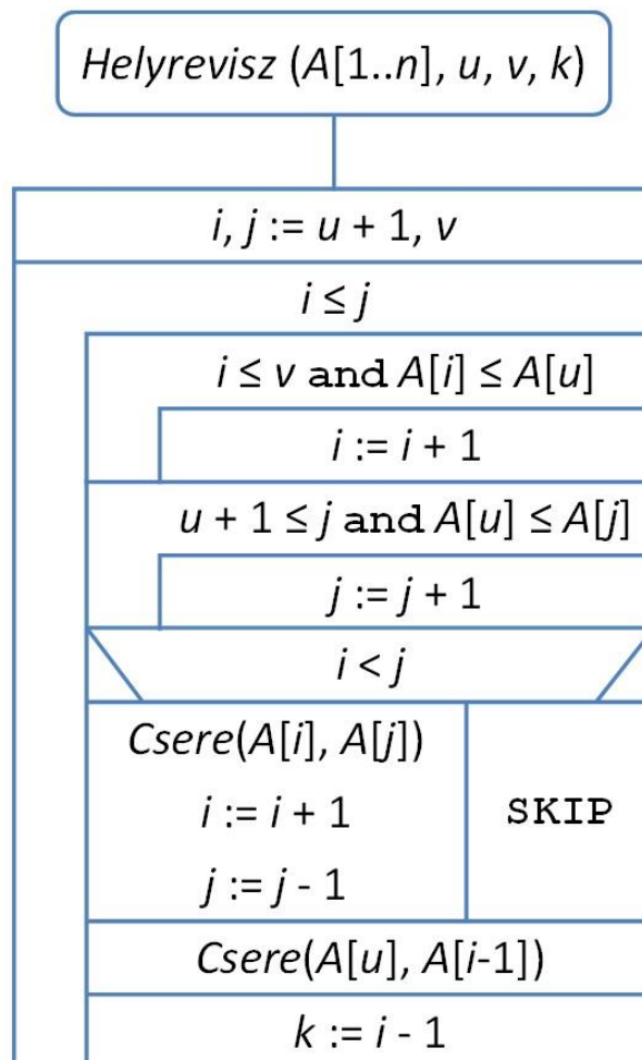
37.3. ábra. Egy elemet a helyére vivő eljárás (a tömb bal szélső elemére)
