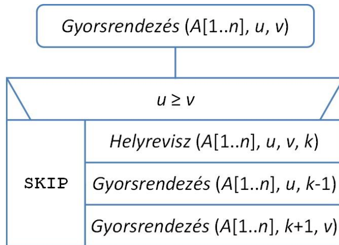
27.2. ábra. A gyorsrendezés rekurzív algoritmus (felső szint)
