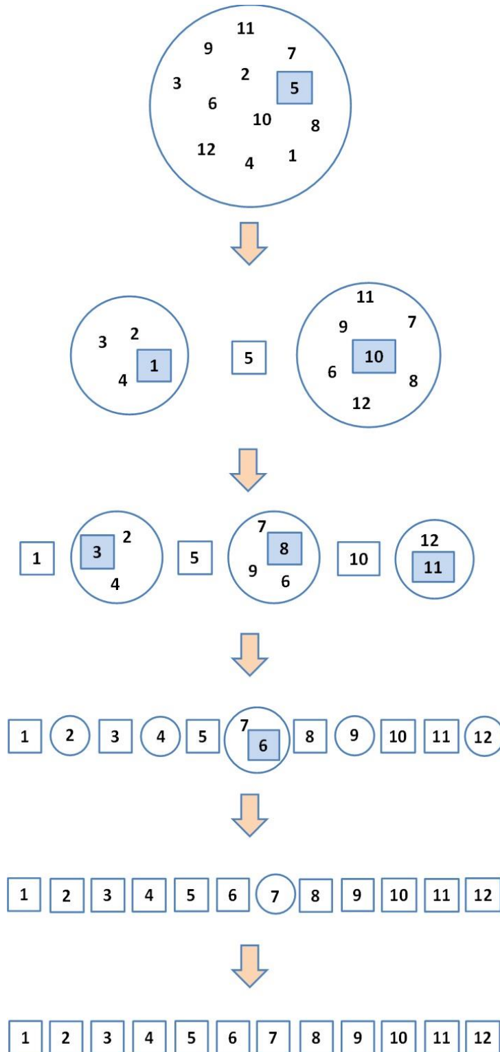
17.1. ábra. A gyorsrendezés elve
