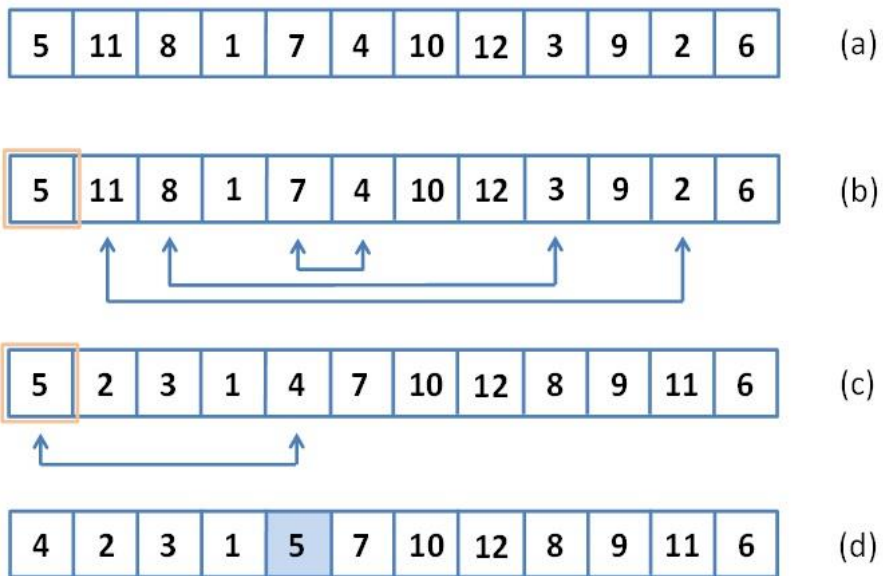
... ... 47.4. ábra. A tömb bal szélső elemének a helyére vitele
