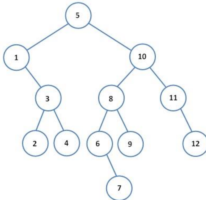
57.5. ábra. A gyorsrendezés egy lehetséges hívási fája
