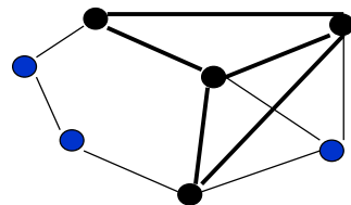
indukált részgráf
