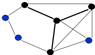
részgráf
