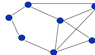
összefüggő
