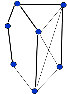
Egy feszítőfa
