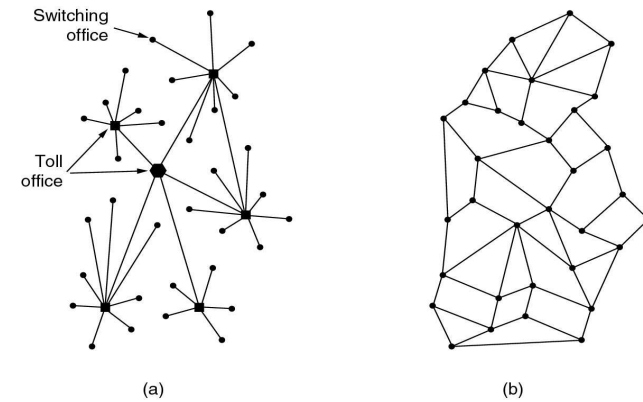
Hierarchikus telefon-hálózat
