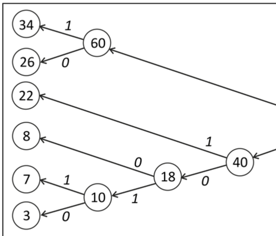
3.1. ábra. A Huffman kód bináris fája
