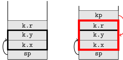
21. ábra. A dynamic_cast működése.
