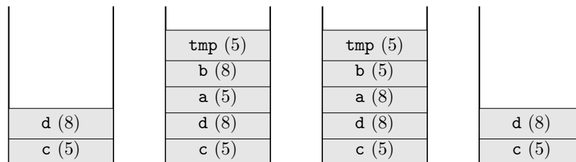
6. ábra. A swapWrong függvény szemléltetése a stack-en.
