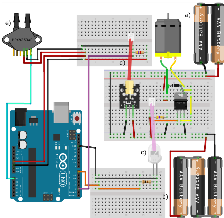
4. ábra: Az Arduino UNO-hoz csatlakoztatott áramkörök megépítése dugaszos próbapaneleken (breadboardokon) 3
